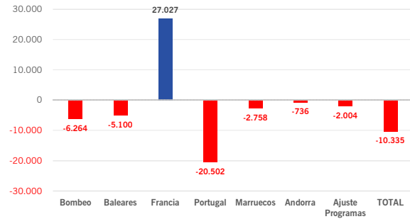
Intercambios y bombeos (media diaria) Septiembre 2019
