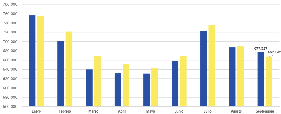
Generación vs Demanda (media diaria) 2019 (MWh)
