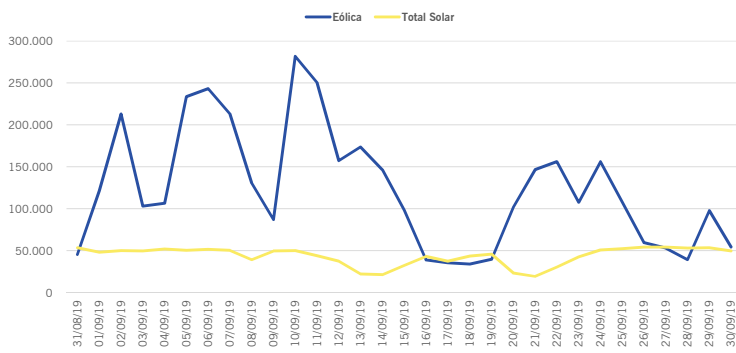
Generación Eólica y Solar Septiembre 2019 (MWh)
