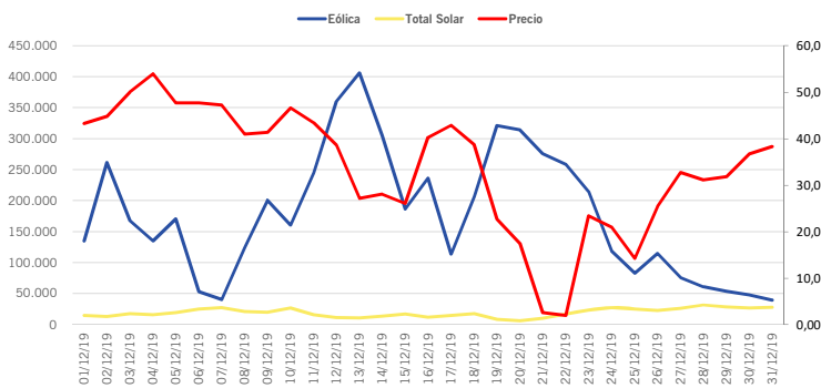
Generación Eólica y Solar Diciembre 2019 (MWh)
