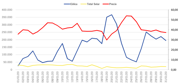
Generación Eólica y Solar Enero 2020 (MWh)
