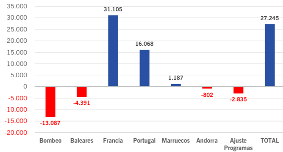
Intercambios y bombeos (media diaria) Enero 2020
