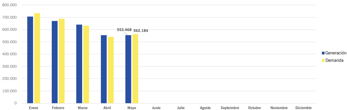
Generación vs Demanda (media diaria) 2020 (MWh)
