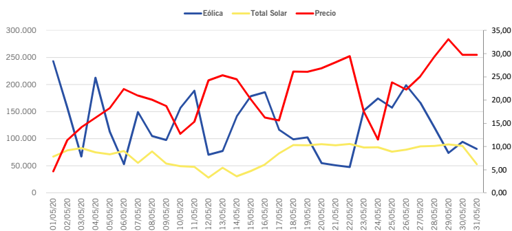
Generación Eólica y Solar Mayo 2020 (MWh)
