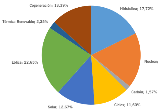
Mix programa Final MAYO-2020
