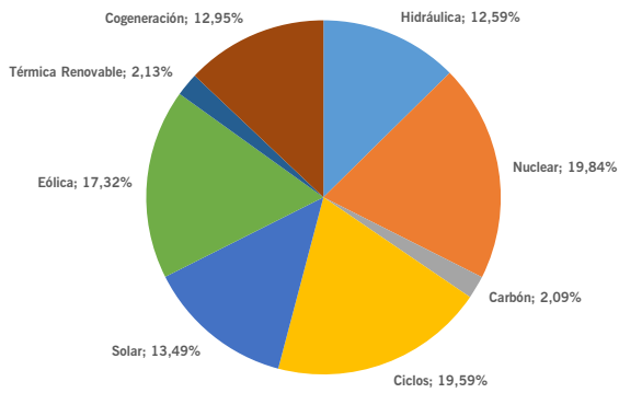
Mix programa Final JUNIO-2020
