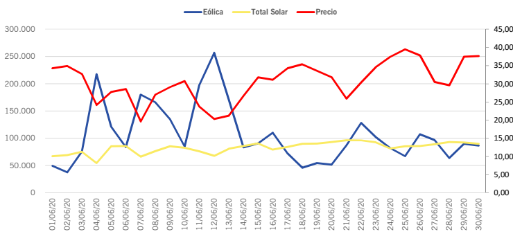
Generación Eólica y Solar Junio 2020 (MWh)
