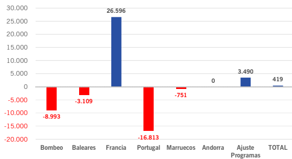
Intercambios y bombeos (media diaria) Junio 2020
