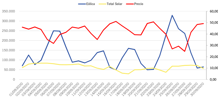
Generación Eólica y Solar Septiembre 2020 (MWh)
