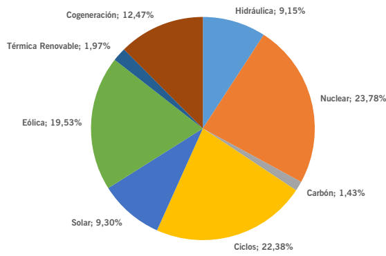
Mix programa Final SEPTIEMBRE-2020
